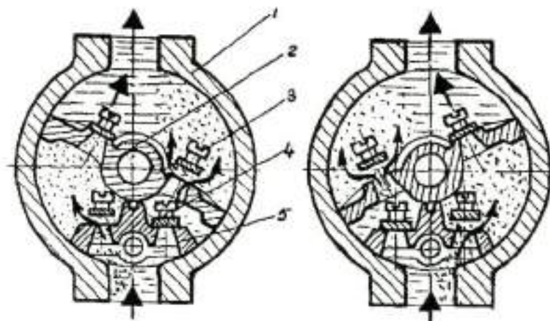
Рис. 5.1. Схема работы насоса
